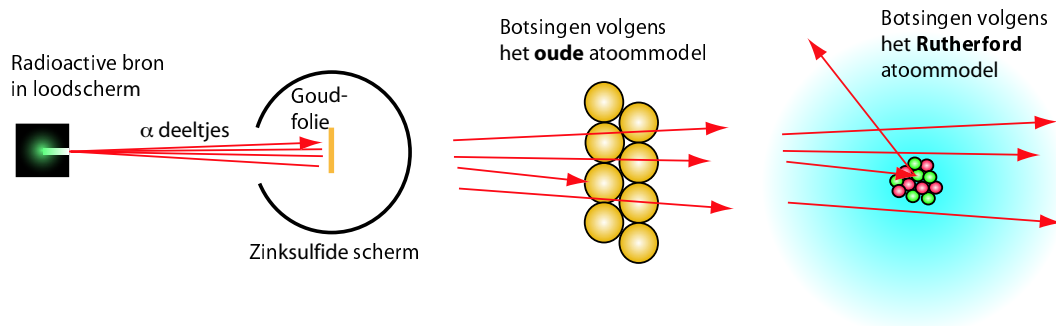
Figuur 6.1: Rutherford verstrooiingsexperiment. In de linker afbeelding is geïllustreerd hoe een bundel van alfa deeltjes uit een radioactieve bron op een trefplaatje wordt geschoten. Rond het trefplaatje staat een scherm van zinksulfide dat oplicht als er een alfa deeltje op botst. Door te kijken waar het scherm oplicht kan de verstrooiingshoek worden gemeten. In de middelste afbeelding staat een illustratie van het idee hoe goudatomen in het folie zijn gestapeld volgens het oude atoommodel. Omdat de meeste alfa deeltjes rechtdoor gaan heeft ieder goudatoom kennelijk een hele luchtige (in dit geval is vacuüm-achtige een beter woord) structuur. In de rechter afbeelding staat schematisch een atoom in de visie van Rutherford. Af en toe botst er een alfa deeltje op een atoomkern en verstrooit dan onder een grote hoek. De meeste alfa deeltjes vliegen door de elektronenwolk rond de kern en worden niet of nauwelijks afgebogen.
