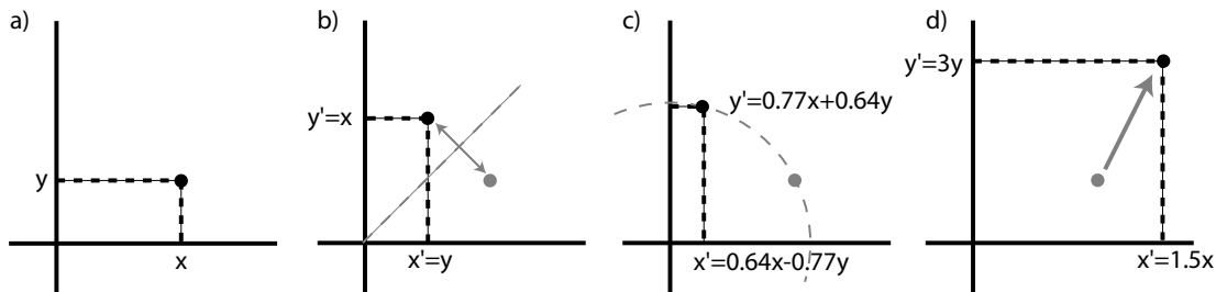
Figuur A.1: Voorbeelden van lineaire transformaties in twee dimensies (ofwel het platte vlak). In figuur a) wordt een punt in het platte vlak uitgebeeld met coördinaten (x, y) . In figuur b) wordt dat punt gespiegeld in een diagonale lijn door de oorsprong. In c) wordt het punt geroteerd over een hoek van 50^\circ tegen de klok in. In d) wordt een willekeurige schaal transformatie uitgevoerd die de lengtes in de x richting met 1.5 vermenigvuldigt en in de y richting met 3.
