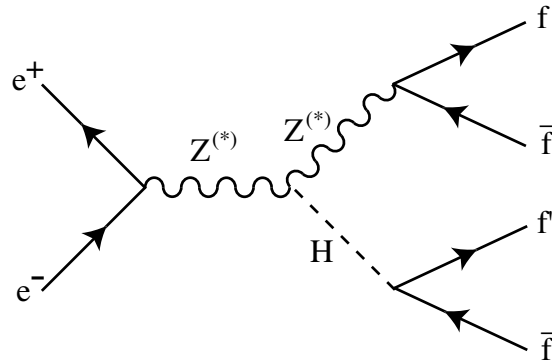
Figuur 10.2: Feynman diagram voor het dominante productieproces van Higgs bosonen bij de LEP versneller.
