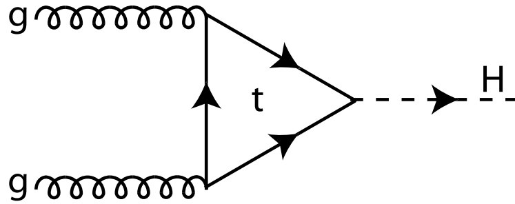
Figuur 10.6: Laagste orde Feynman diagram voor Higgs productie door gluon fusie.
